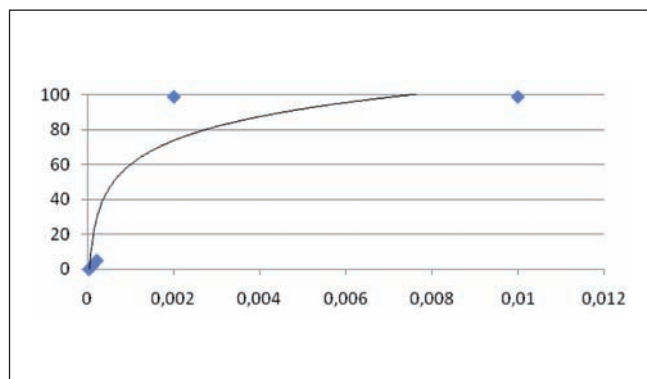
FIGURA 8. Estudi de la reacció de \beta -boració d'etil crotonat amb coure (conversió/mmols de Cu).
